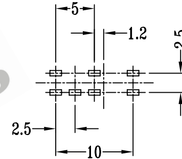
P.C.B LAYOUT
